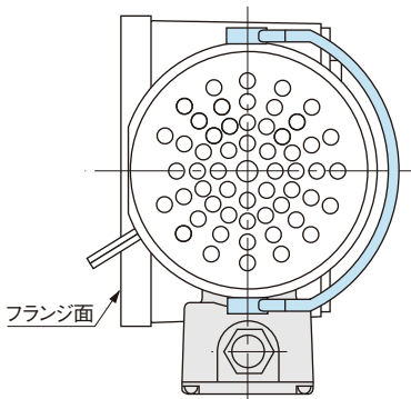
モータ容量別寸法 G3・H2・F・F3シリーズ共通
