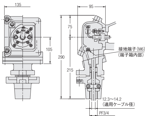
安全増防爆形 端子箱詳細図・保護管方式
